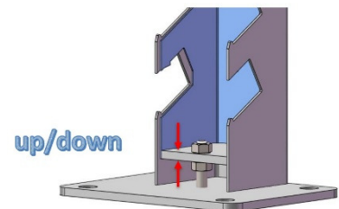
Patentierter Spannvorrichtung
